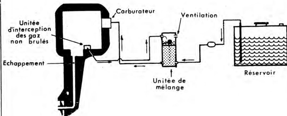
SYSTÈME ANTI-POLLUTION
